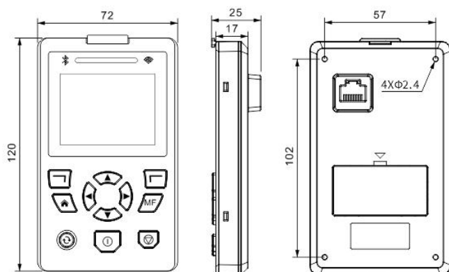
图 C-4 LCD 外引键盘安装尺寸（单位：mm）
