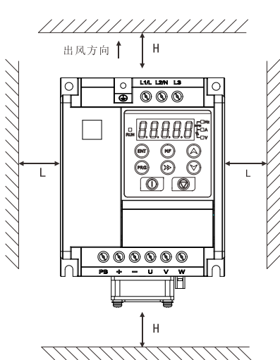
图 2-1 安装的间隔距离
