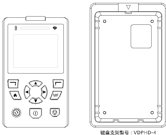
图 7-3 LCD 键盘及其安装支架
