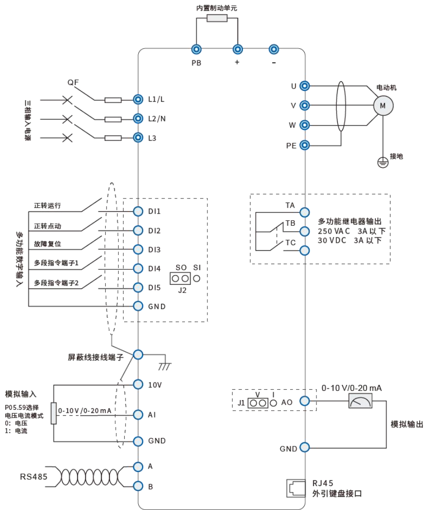
图 2-6 M100 系列变频器系统配线图
