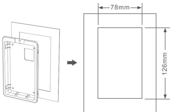
图 C-5 双显外引键盘支架安装尺寸 (单位: mm)
