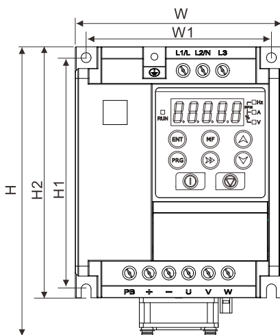
图 2-4 壁挂式安装示意图
