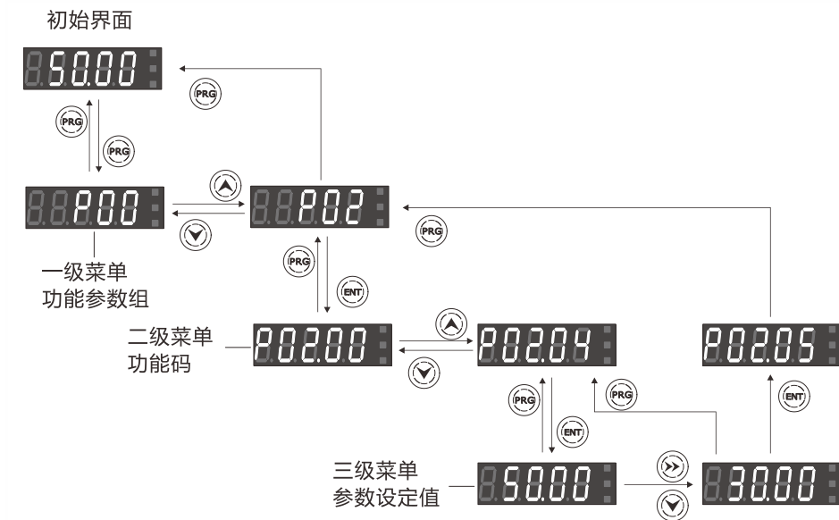
图 3-2 参数查询与修改流程
