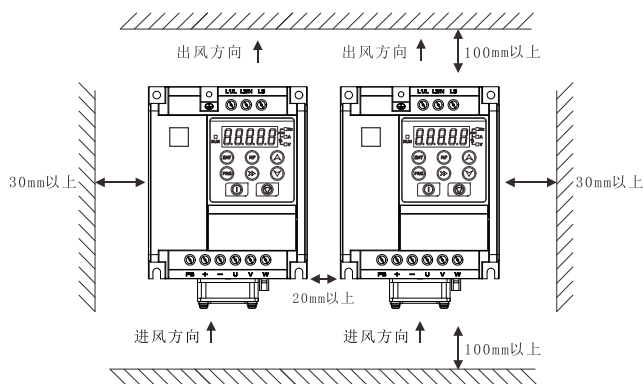
图 2-3 两台变频器左右安装
